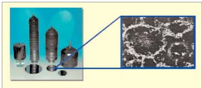
Abb. 5 Vergrößerung eines Galliumarsenid (GaAs)-Halbleiters (»Schäfchen-Bild«): Kleine flüssige GaAs-Tröpfchen (hell) im GaAs-Kristall (dunkel) beeinflussen die Eigenschaften des Halbleiters negativ.
